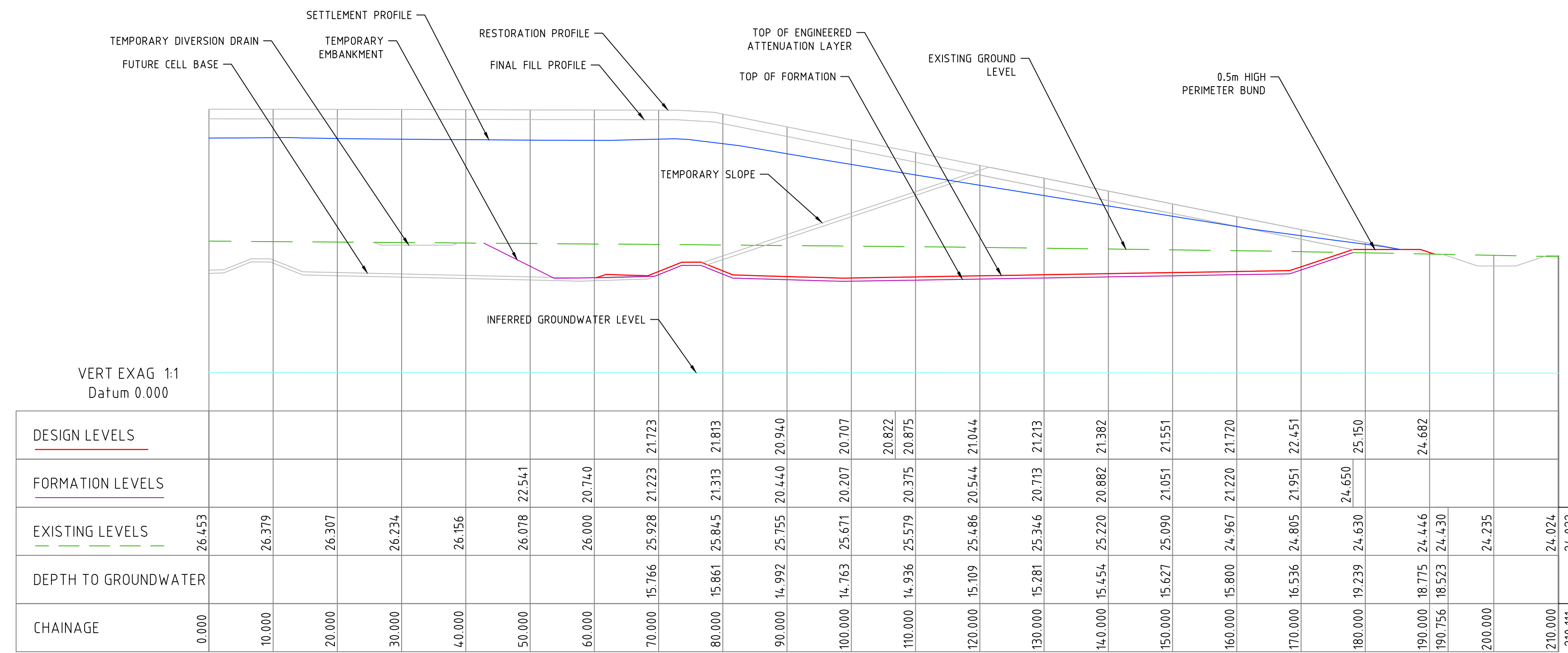
B LONG SECTION CELL 1 SCALE: 1:500
