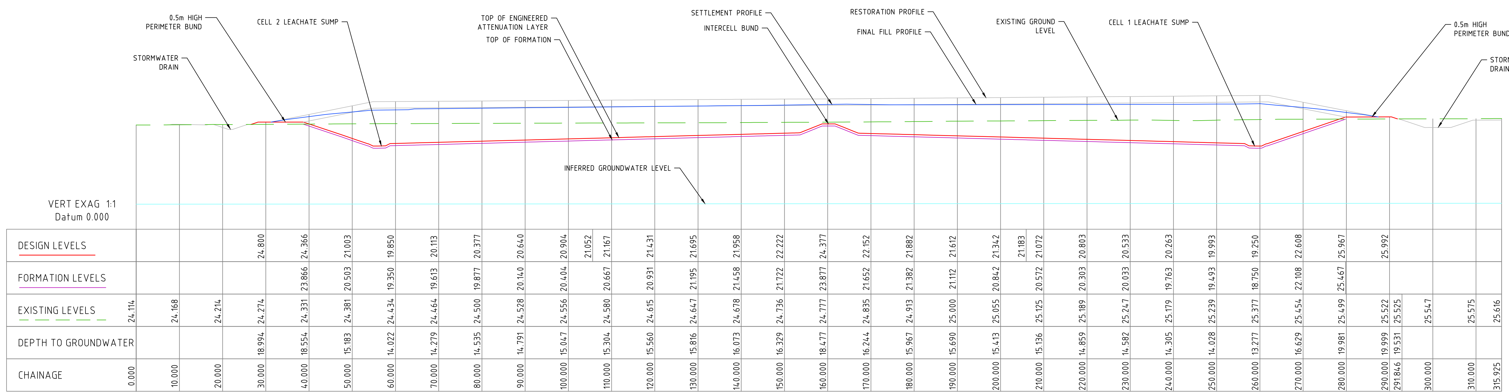
C LONG SECTION CELL 1 & CELL 2 SCALE: 1:500
